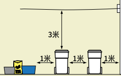
側面圖
